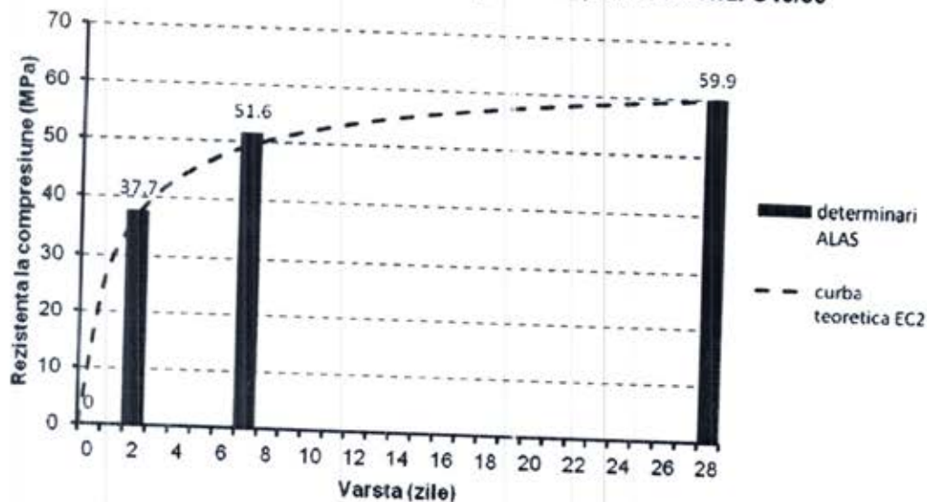
Evolutia rezistentei la compresiune pentru betonul C40/50
